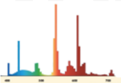
lückenhaftes Lichtspektrum einer Energiesparlampe
